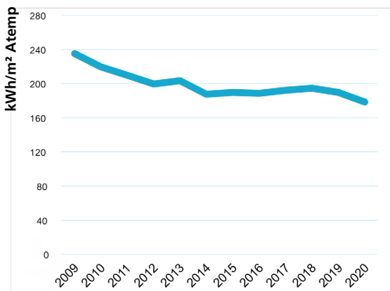
FIGUR 20. Energi användning (normalårskorrigerad) per kvadratmeter. Källa: Teknik- och fastighetsförvaltningen
