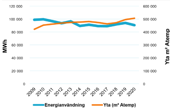
FIGUR 18. Total energianvändning för uppvärmning (normalårskorrigerad) och övrig el (verksamhet och fastighetsel) i förhållande till uppvärmd yta (m² Atemp). I början av perioden gjordes en aktiv satsning på energi-effektivisering och energianvändningen minskade trots att fastighetsbeståndet växte. I slutet av perioden följer energianvändningen utökningen av lokalyta. Källa: Teknik- och fastighetsförvaltningen
