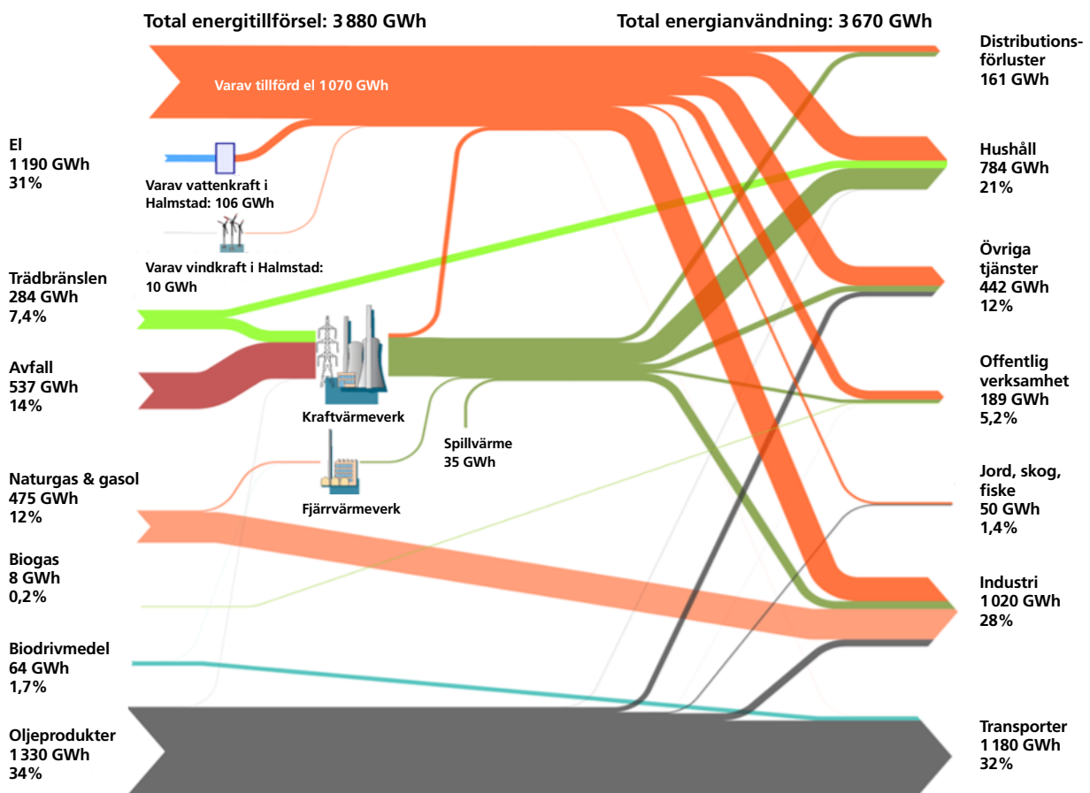
FIGUR 2. Sankey-diagram visar energiflöden i Halmstad baserade på SCB:s statistik år 2012 som redovisades i Halmstads energiplan från 2015 Handlingsprogram för hållbar energi. Källa: Länsstyrelsen i Halland
