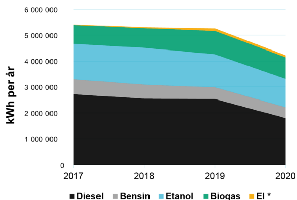
FIGUR 12. Beräknad använd energi per drivmedelstyp i kommunens fordonspark. Bolagens fordon ingår inte. 2020 märks en tydlig pandemieffekt av minskade tjänsteresor.
