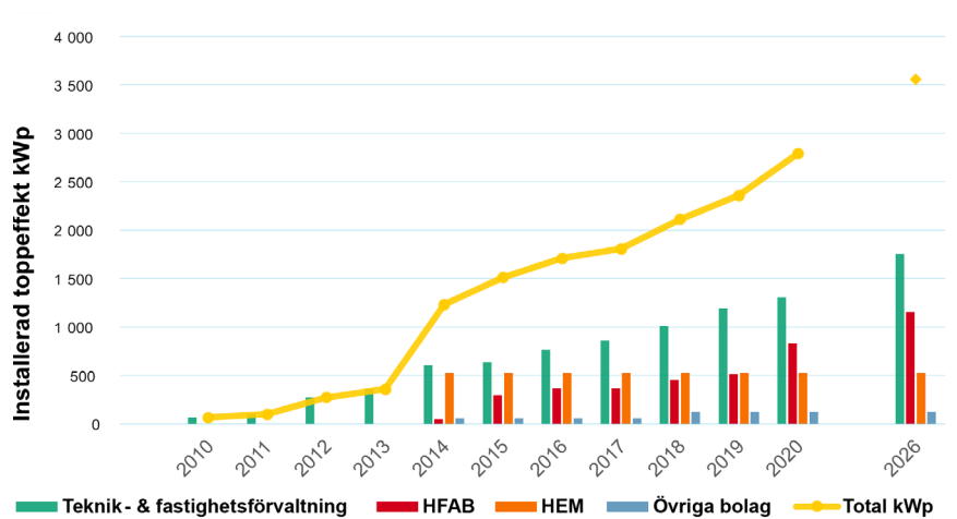
FIGUR 23. Installerad effekt från solceller på kommunala fastigheter perioden 2010–2020 samt redan planerade anläggningar fram till 2026. Samtliga anläggningar är placerade på kommunala tak med undantag av Halmstads Energi och Miljö AB:s markbaserade anläggning på Skedaladeponin. Övriga bolag är Laholmsbuktens VA AB och Halmstad City Airport. Källa: Teknik- och fastighetsförvaltningen, HFAB, HEM
