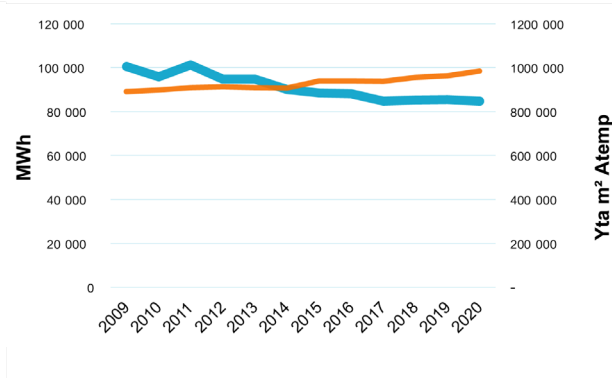
FIGUR 18. Total energianvändning för uppvärmning (normalårskorrigerad) och övrig el (verksamhet och fastighetsel) i förhållande till uppvärmd yta (m² Atemp). I början av perioden gjordes en aktiv satsning på energi-effektivisering och energianvändningen minskade trots att fastighetsbeståndet växte. I slutet av perioden följer energianvändningen utökningen av lokalyta. Källa: Teknik- och fastighetsförvaltningen
