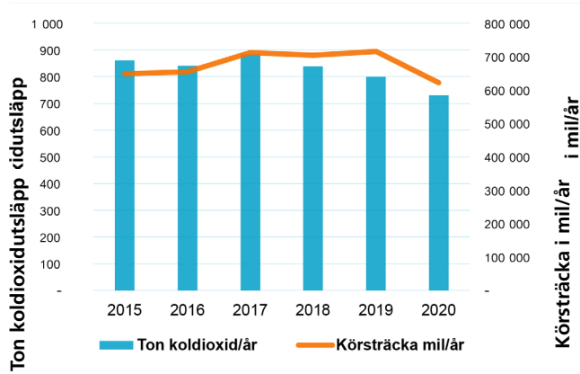
FIGUR 14. Ton koldioxidutsläpp från kommunens fordonspark. Utsläppen minskar något samtidigt som körsträckan har ökat. Bolagens fordon ingår inte. 2020 märks en tydlig pandemieffekt av minskade tjänsteresor. Källa: Halmstads kommuns fordonstatistik
