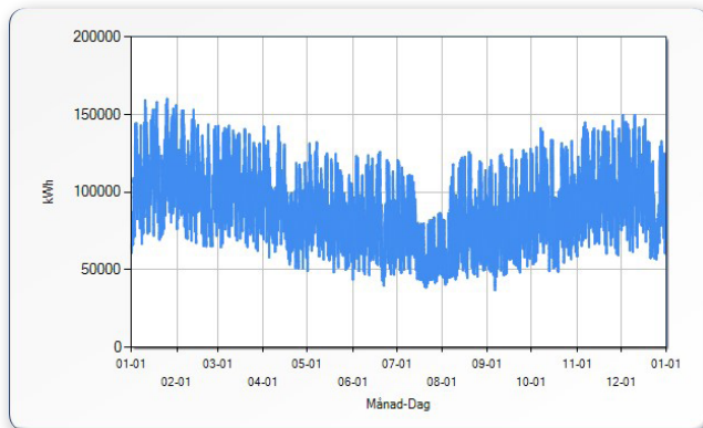
FIGUR 22. Diagrammet visar hur effektuttaget varierar både över året och under dygnet år 2019. Nattetid är effektuttaget lägre, men vinterdagar med låga temperaturer nattetid så kan uttaget vara högt även då. Källa: Halmstad Energi och Miljö AB
