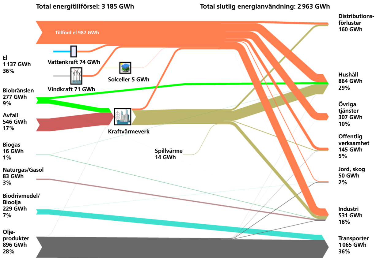
FIGUR 1. Sankey-diagram visar energiflöden i Halmstad baserade på SCB:s statistik år 2018. Källa: Länsstyrelsen i Halland
