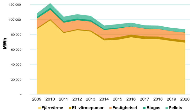
FIGUR 17. Användning av olika energislag i allmännyttans bostadsbestånd. Hushållens el är inte inkluderat, endast el för driftfastighetens gemensamma funktioner, såsom trapphus och gemensamma tvättstugor redovisas som fastighetsel. Elen är förnybar. El- och värmepumpar redovisas separat. HFAB har sedan tidigare fasat ut oljepannor med fossila bränslen. Fjärrkyla används inte. Källa: HFAB
