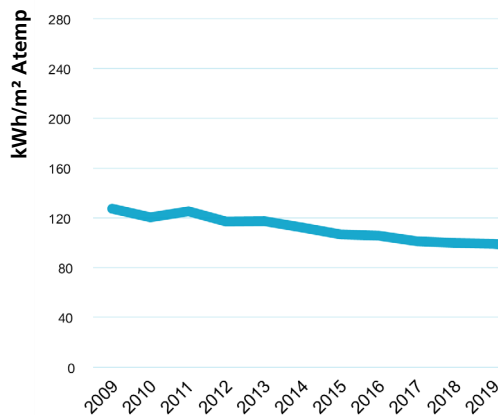
FIGUR 20. Energi användning (normalårskorrigerad) per kvadratmeter. Källa: Teknik- och fastighetsförvaltningen
